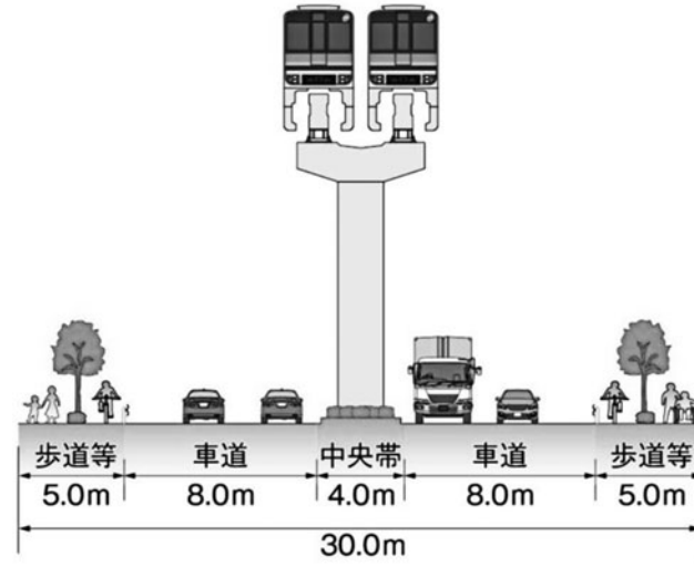
新青梅街道標準横断面図
